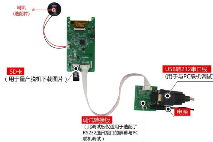
图 1-3 调试工具图
