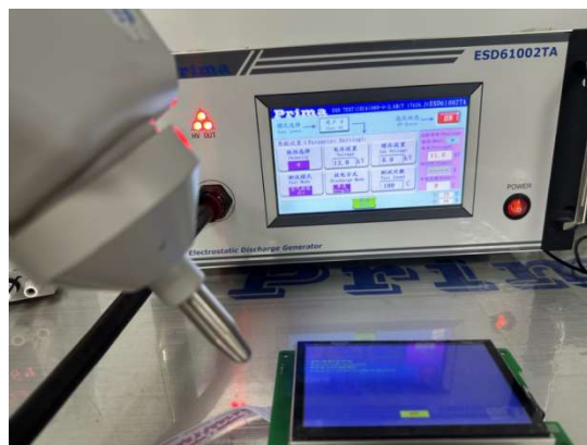
图 4-2 ESD 测试图
