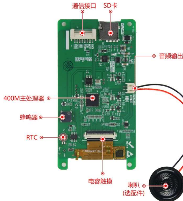
图 1-2 硬件配置图
